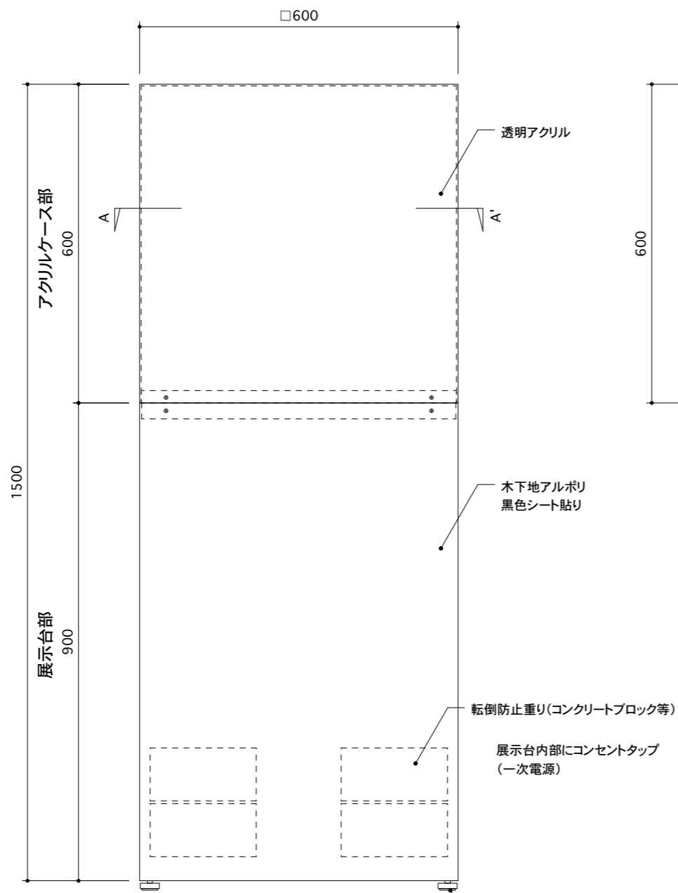
側面図
