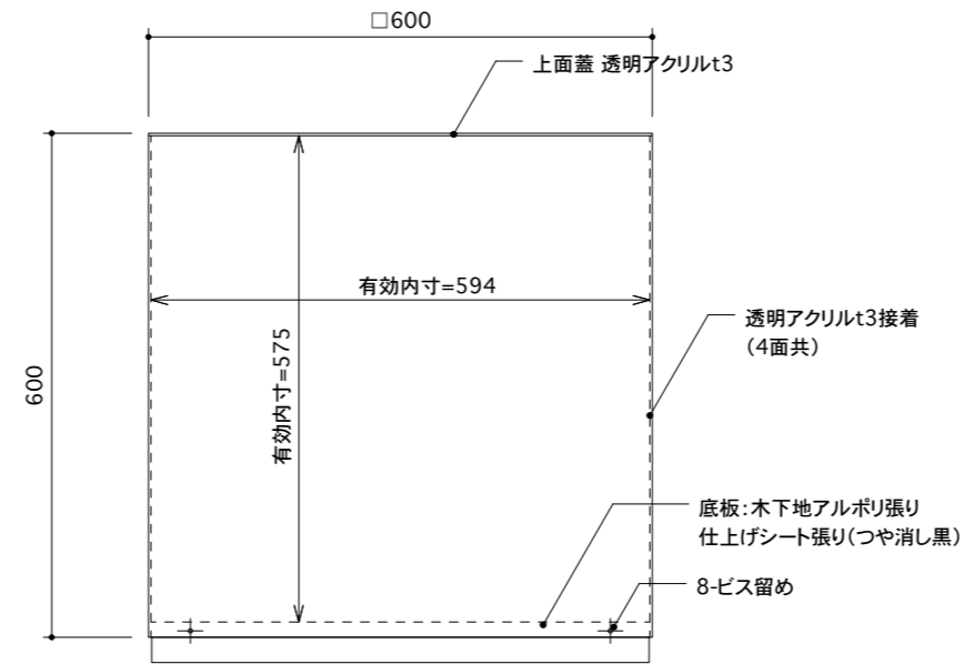
アクリルケース部側面図
